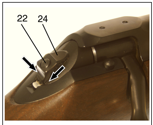
Abb. 12 // Waffe gesichert
