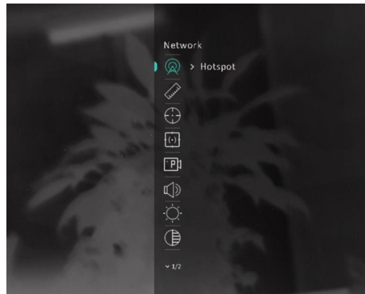
Abbildung 2-7 Hauptmenü
