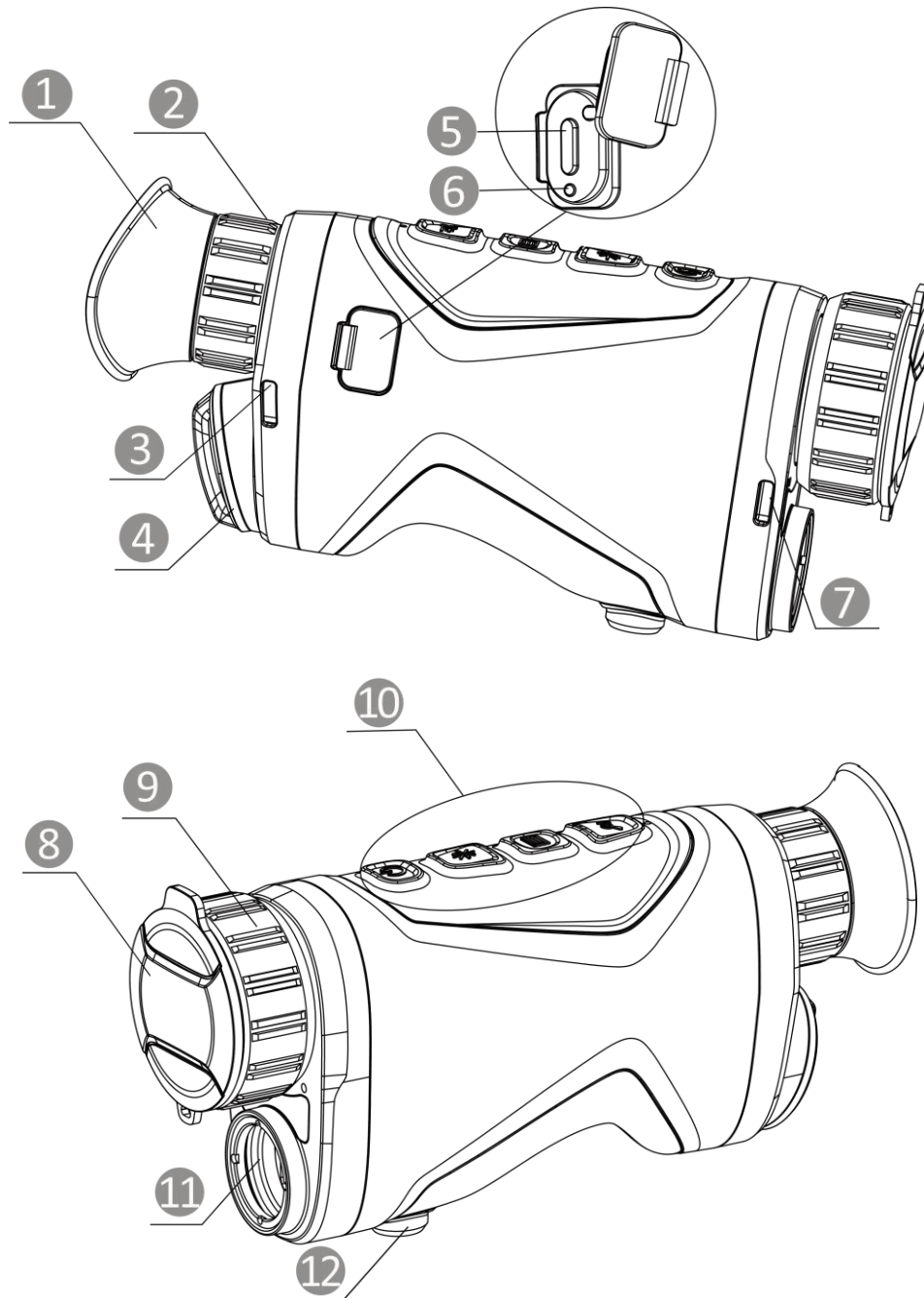
Abbildung 1-1 Aufbau
